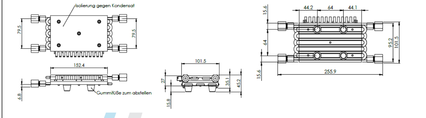
Abmessungen / Befestigung / Anschlüsse
