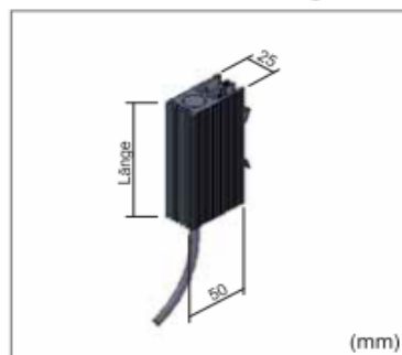
Maßzeichnung
