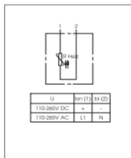
Schaltbild
