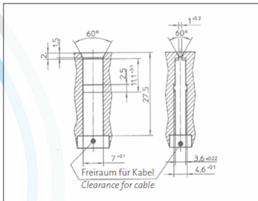
Gehäuse Gegenstecker 6,3 x 0,8 mm
