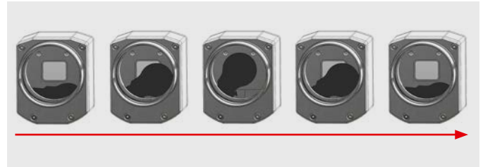
Zur Offsetreferenzierung wird in das Gesichtsfeld des Infrarot-Sensorarrays kurzzeitig eine Temperaturreferenz hineinbewegt.
